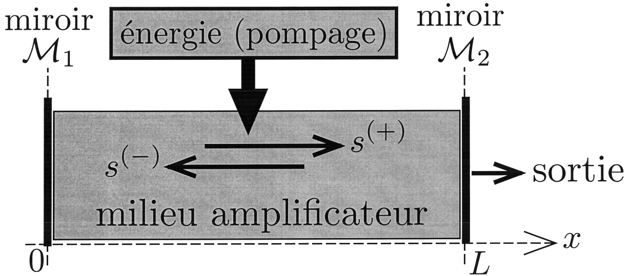
Figure 5: Représentation schématique d'une cavité laser composée d'un milieu amplificateur de lumière compris entre deux miroirs.
