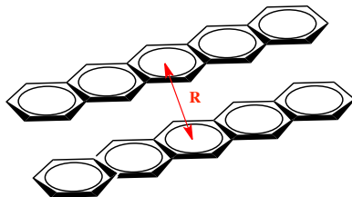
Figure 3 – Dimère “sandwich” du pentacène, caractérisé par une distance de séparation R .
